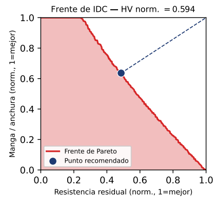
Figura 5: Frente de Pareto de IDC (resistencia frente a manga, esto es la relación eslora/manga L/B , a Froude fijo). Cada eje se normaliza respecto al propio rango del frente (1 = mejor); el área sombreada es el hipervolumen normalizado ( \approx 0,59 ). Se aprecian el compromiso entre ambos objetivos y la rodilla en la que se sitúa el punto recomendado (azul), unido al punto utópico.
