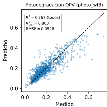
Figura 3: Bondad de ajuste del sustituto de OpenNN (8 neuronas) para la fotodegradación de la mezcla OPV: R^2 = 0,77 sobre las 1040 mezclas ( R^2 = 0,80 en el conjunto de test).
