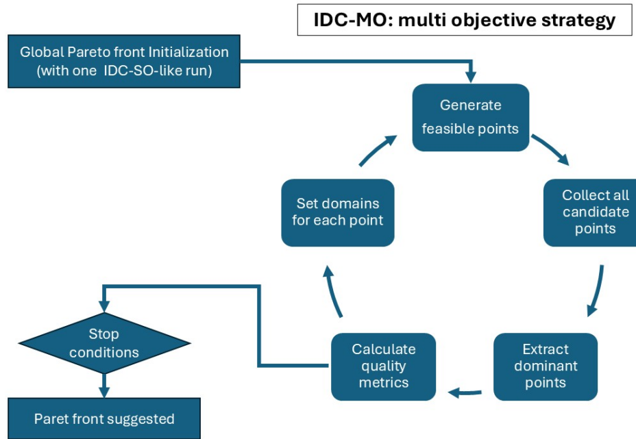
Figura 2: Estrategia multiobjetivo de IDC (IDC-MO): se inicializa el frente de Pareto global (una corrida tipo IDC-SO) y, para cada punto del frente, se generan puntos factibles, se recopilan los candidatos, se extraen los dominantes y se calculan métricas de calidad hasta la parada.
