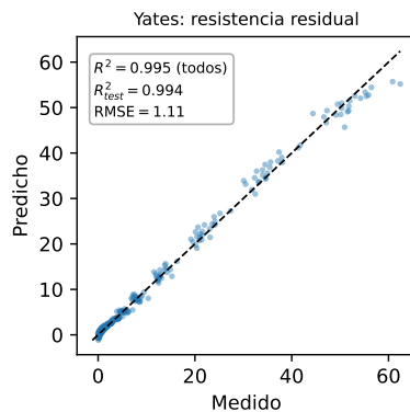
Figura 4: Bondad de ajuste del sustituto de OpenNN para la resistencia residual del velero (4 neuronas): R^2 = 0,995 sobre las 308 medidas ( R^2 = 0,99 en el conjunto de test).
